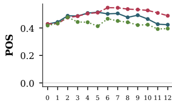
Base GPT-2
